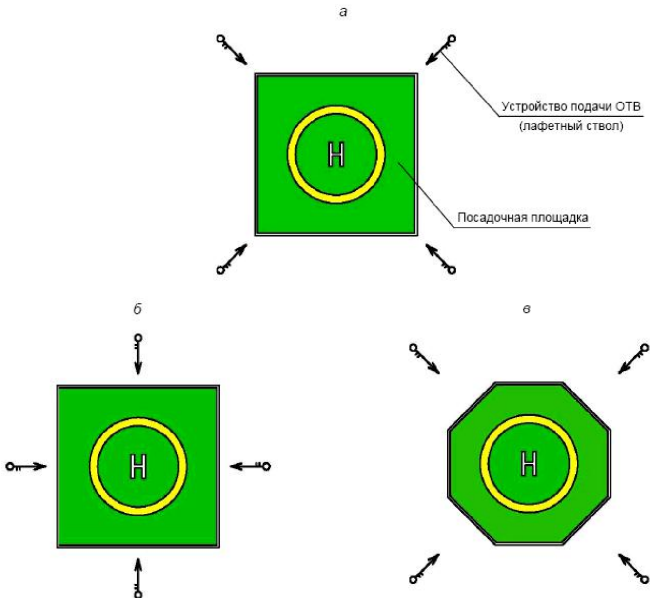
а - диагональное ; б - линейное; в - радиальное Рисунок А.1 - Схемы размещения стационарных лафетных стволов
